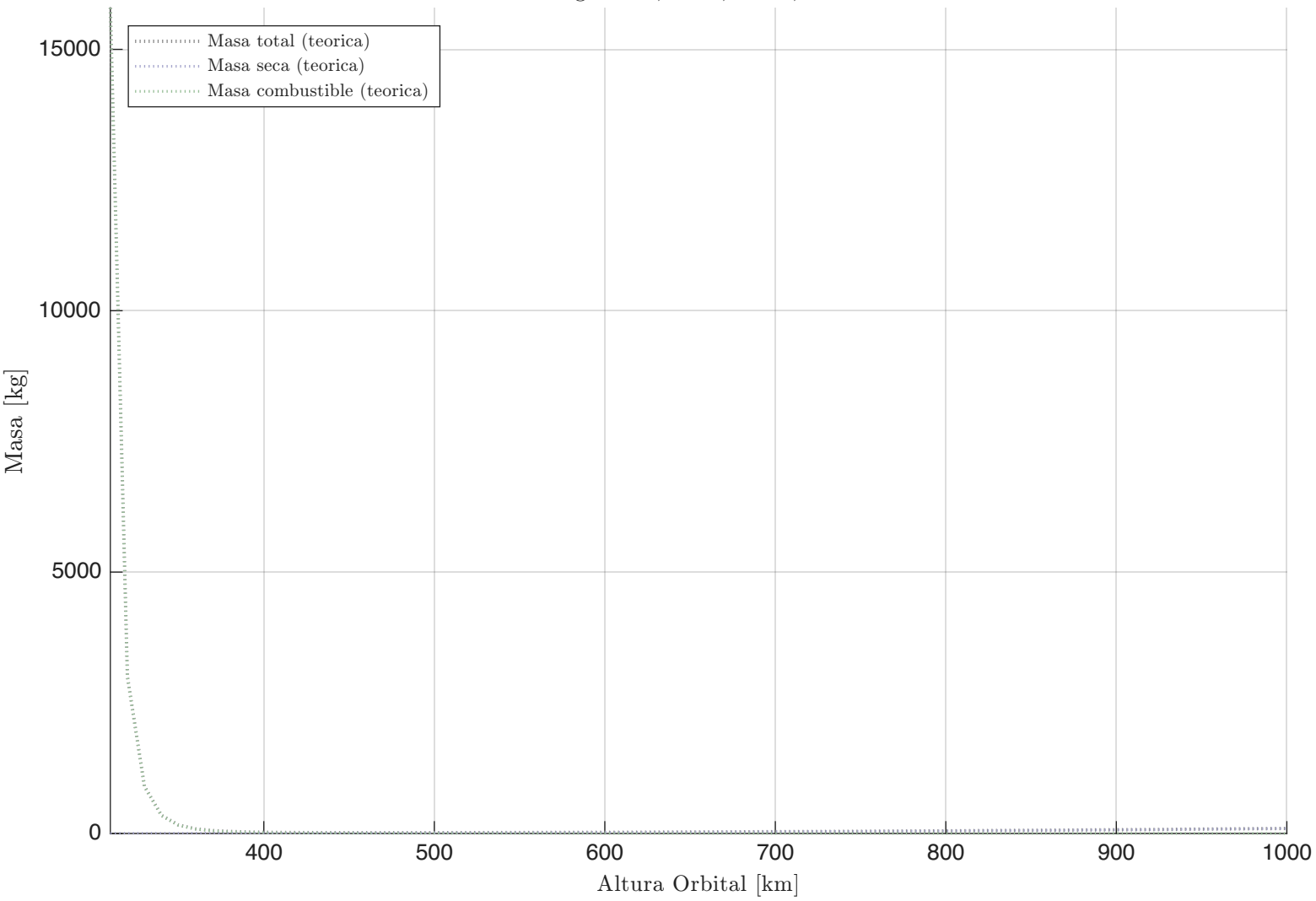
Desglose de Masas vs. Altura Config: 2 Sat, 2 Tel, Det 1, Korsch
